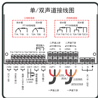
单、双声道接线图
